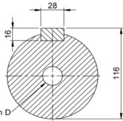
KESİT A-A
